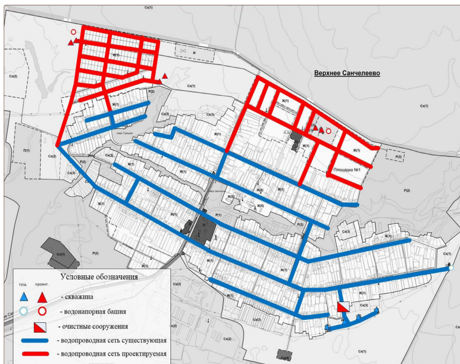
Рисунок 2.4.9.1 – Расположение существующих и перспективных объектов системы водоснабжения с. Верхнее Санчелеево
