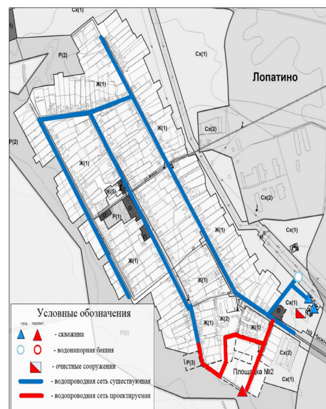
Рисунок 2.4.9.2 – Расположение существующих и перспективных объектов системы водоснабжения с. Лопатино
